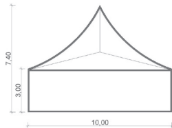
Seitenansicht
