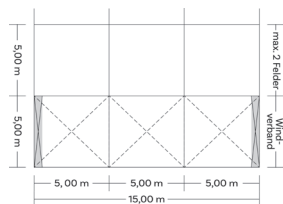
Draufsicht
