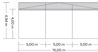
Seitenansicht
