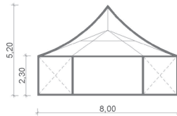
Seitenansicht
