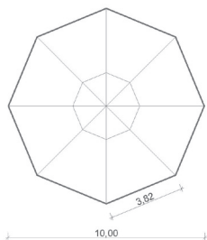
Draufsicht
